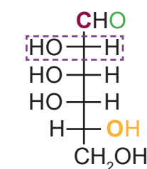
D-Talose
