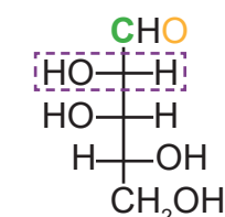
D-Lyxose
